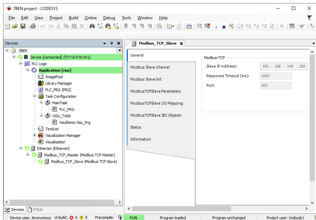
Fig. 61: Modbus TCP communication
