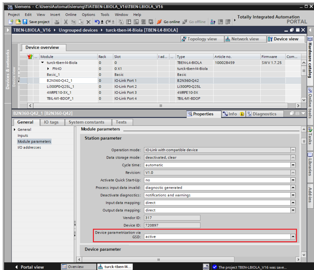
Fig. 90: Example: TIA Portal, "Device parameterization via GSD" parameter
