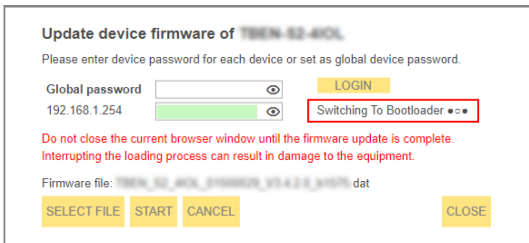
Fig. 115: Firmware update progress
